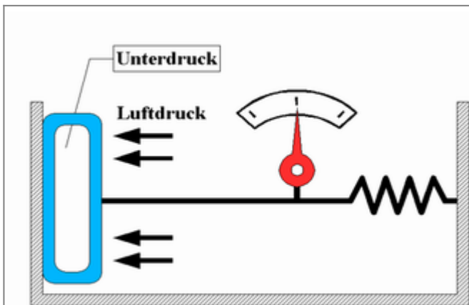
Abb. 3: Funktionsprinzip eines Dosenbarometers
